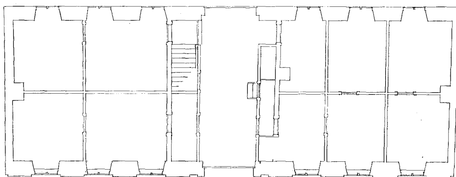
Elers' Collegium. Etageplaner. Nederst: Stueetagen, derover 1. Sal og 2. Sal. Opmaalinger, 1:200, af Preben Geismar, O. Hagen, Holger Sørensen 1934.
