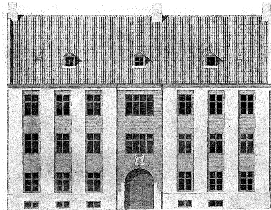
Elers' Collegium. Façade mod St. Kannikestræde. Opmaaling, 1 : 200, af Preben Geismar 1934.
