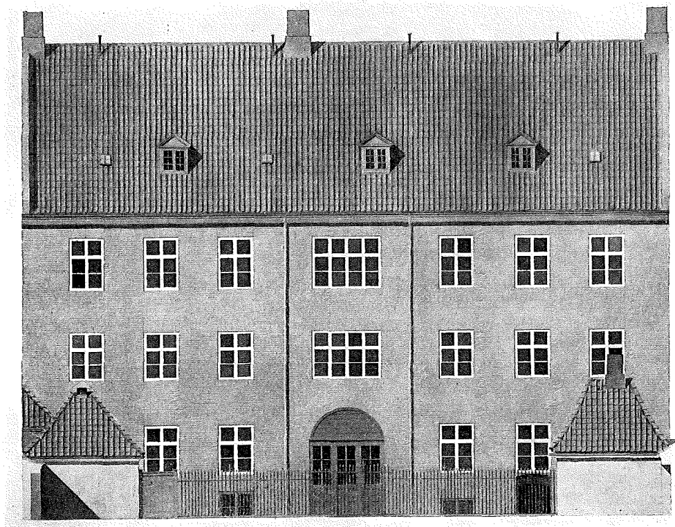
Elers' Collegium. Façade mod Gaard og Have. Opmaaling, 1:200, af Holger Sørensen 1934.
